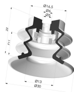
Ventouse 2.5 Soufflets Série 96C Ø 30MM
