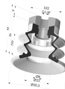
Ventouse 2.5 Soufflets Série 96C Ø 50MM
