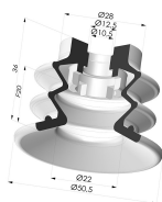
Ventouse 2.5 Soufflets Série 96C Ø 50MM
