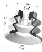
Ventouse 2.5 Soufflets Série 96C Ø 50MM
