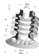
Ventouse 4.5 Soufflets Série 95-2 Ø 41MM
