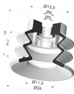
Ventouse 2.5 Soufflets Série 96C Ø 25MM
