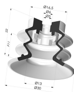
Ventouse 2.5 Soufflets Série 96C Ø 30MM
