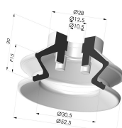
Ventouse 1.5 Soufflets Série 97B Ø 52.5MM
