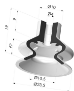
Ventouse 1.5 Soufflets Série 1 Ø 23MM - à Décrochement
