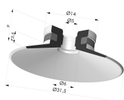
Ventouse Plate Série 9 Ø 31.5MM Référence produit : 9 30-- A
