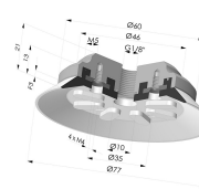
Ventouse Plate Série 90 Ø 75MM
