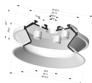
Ventouse 1.5 Soufflets Série 91 Ø 159,5MM
