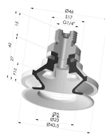
Ventouse 1.5 Soufflets Série 91 Ø 40MM
