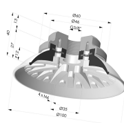
Ventouse Plate Série 94 Ø 100MM
