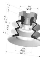
Ventouse 2.5 Soufflets Série 96 Ø 52MM
