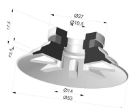
Ventouse Plate Série 90 Ø 53MM
