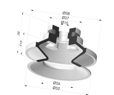
Ventouse 1.5 Soufflets Série 91 Ø 50MM Référence produit : 91 50-- A
