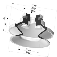
Ventouse 1.5 Soufflets Série 91 Ø 50MM Référence produit : 91 50-- A
