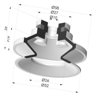
Ventouse 1.5 Soufflets Série 91 Ø 50MM
