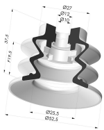
Ventouse 2.5 Soufflets Série 96 Ø 52MM
