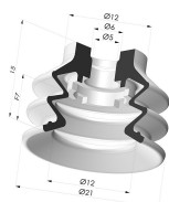
Ventosa 2.5 Soffietti Serie 96C Ø 20MM
