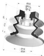
Ventosa 2.5 Soffietti Serie 96C Ø 40MM
