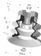
Ventosa 2.5 Soffietti Serie 96C Ø 50MM
