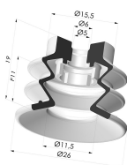
Ventosa 2.5 Soffietti Serie 96C Ø 25MM
