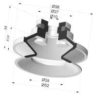
Ventosa 1.5 Soffietti Serie 91 Ø 50MM
