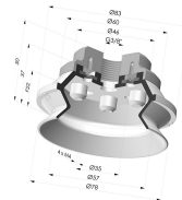
Ventosa 1.5 Soffietti Serie 91 Ø 75MM
