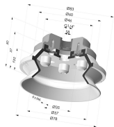
Ventosa 1.5 Soffietti Serie 91 Ø 75MM
