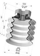
Ventosa 4.5 Soffietti Serie 92 Ø 50MM
