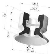
Ventosa Piatta Serie PFG Ø 10.5 mm
