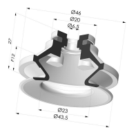
Ventosa 1.5 Soffietti Serie 91 Ø 40MM Riferimento prodotto: 91 40-- A
