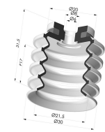
Ventosa 4.5 Soffietti Serie 92 Ø 30MM
