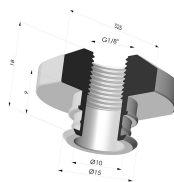
Inserto a resca Femmina G1/8"
