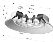
Ventosa Piatta Serie PFG Ø 116.5 mm
