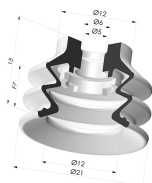
Ventosa 2.5 Fole Série 96C Ø 20MM
