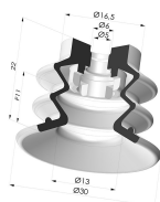
Ventosa 2.5 Fole Série 96B Ø 30MM
