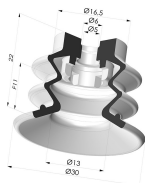
Ventosa 2.5 Fole Série 96C Ø 30MM
