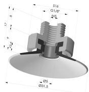
Ventosa plana Série 9 Ø 31,5 mm
