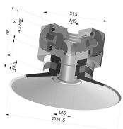
Ventosa plana Série 9 Ø 31,5 mm
