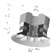
Ventosa plana Série 90 Ø 22 mm
