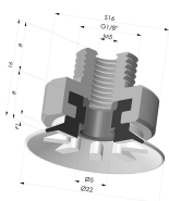
Ventosa plana Série 90 Ø 22 mm
