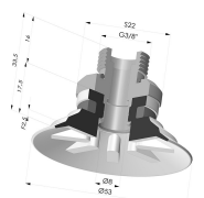
Ventosa plana Série 90 Ø 53 mm
