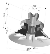
Ventosa plana Série 90 Ø 53 mm
