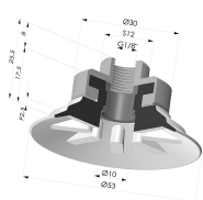
Ventosa plana Série 90 Ø 53 mm
