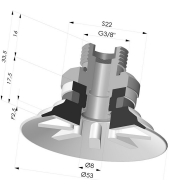
Ventosa plana Série 90 Ø 53 mm
