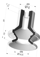
Ventosa 1.5 Fole Série 91 Ø 16,5 mm
