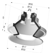
Ventosa 1.5 Fole Série 91 Ø 31,8 mm
