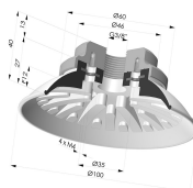
Ventosa plana Série 94 Ø 100 mm
