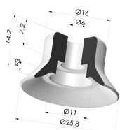
Ventosa plana da série PFG Ø 25,8 mm
