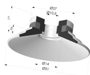
Ventosa plana Série 9 Ø 51 mm
