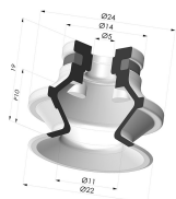
Ventosa 1.5 Fole Série 91 Ø 22,2 mm
