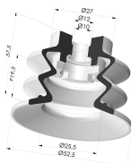
Ventosa 2.5 Fole Série 96 Ø 52MM
