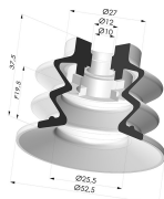
Ventosa 2.5 Fole Série 96 Ø 52MM
